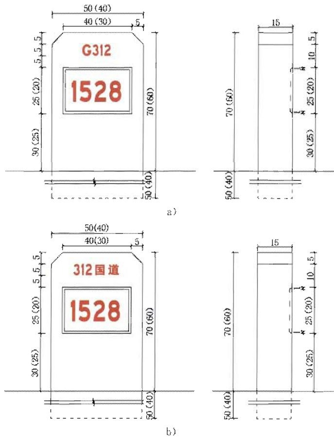
图 245 里程碑
