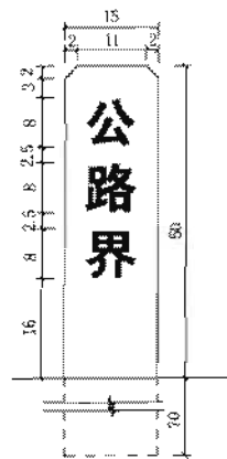
图 248 公路界碑
