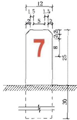
图 247 百米桩
