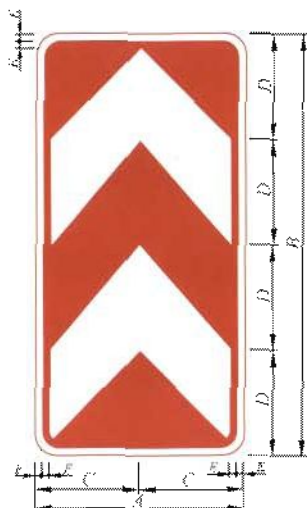
图 242 路 38 两侧通行
